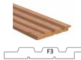
Maatvoering model F3
