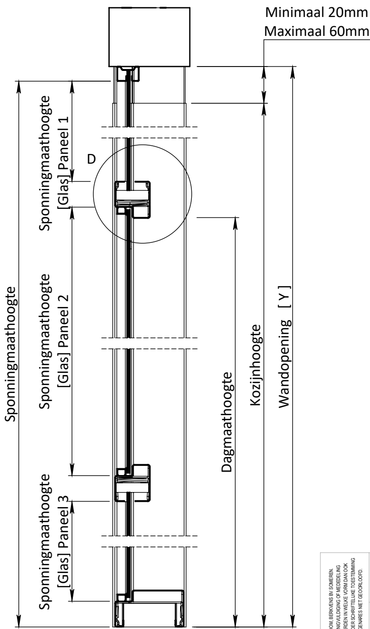
DOORSNEDE B-B
