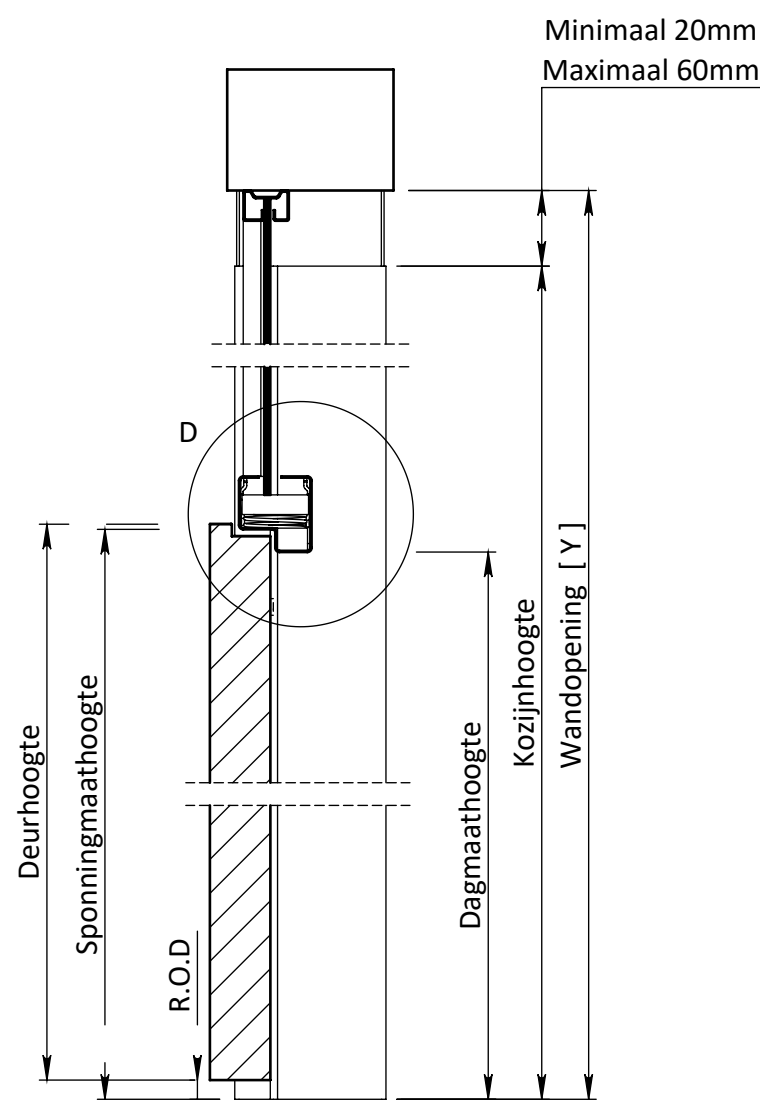
DOORSNEDE B-B
