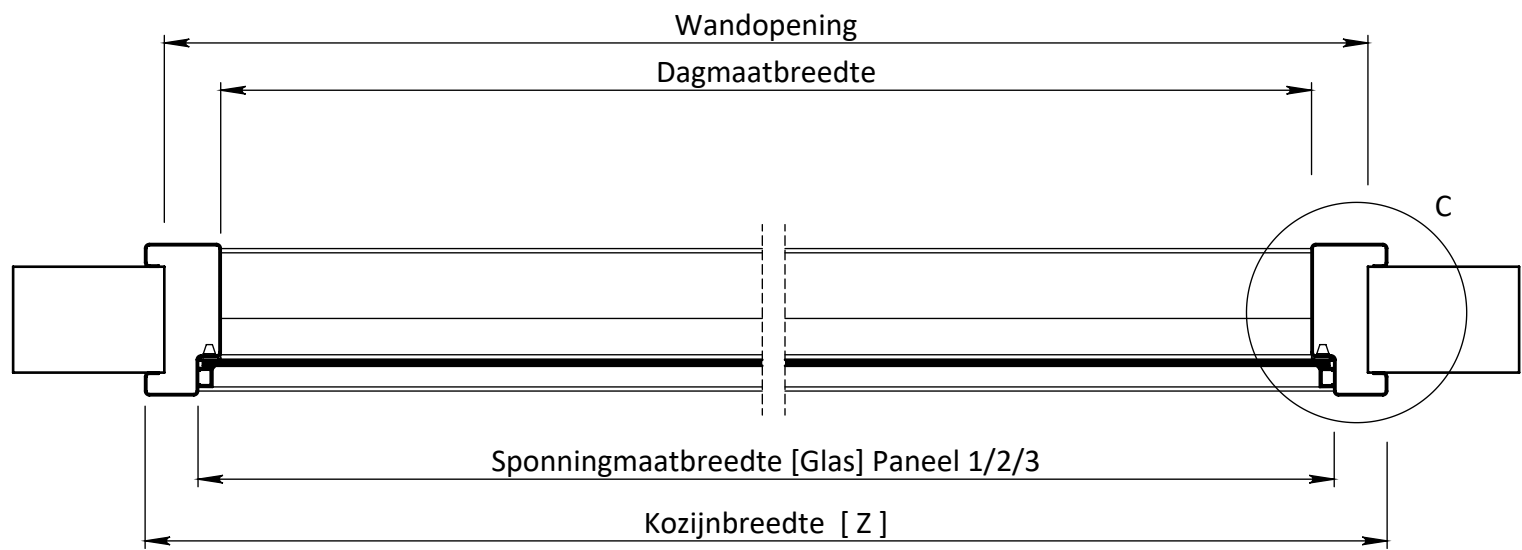
DOORSNEDE A-A
