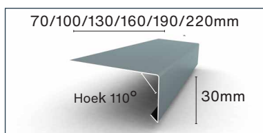
6. Alu raamdorpelprofiel
