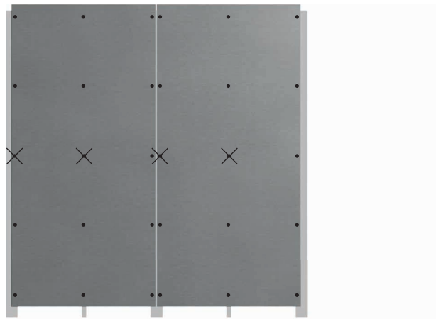
Voorbeeld: Verticaal gemonteerde panelen met één aluminium tussenprofiel
