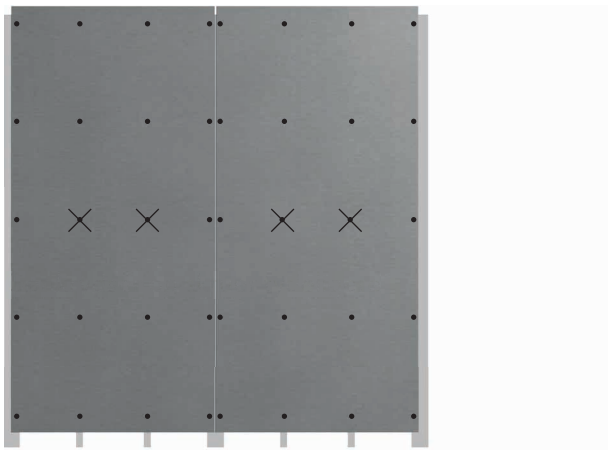
Voorbeeld: Verticaal gemonteerde panelen met twee aluminium tussenprofielen
