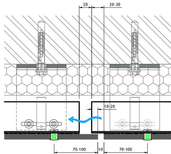
Horizontale doorsnede over plafond
