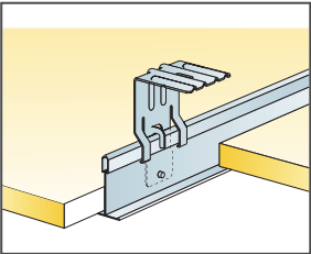
Ophanging met Connect Ophangbeugel
