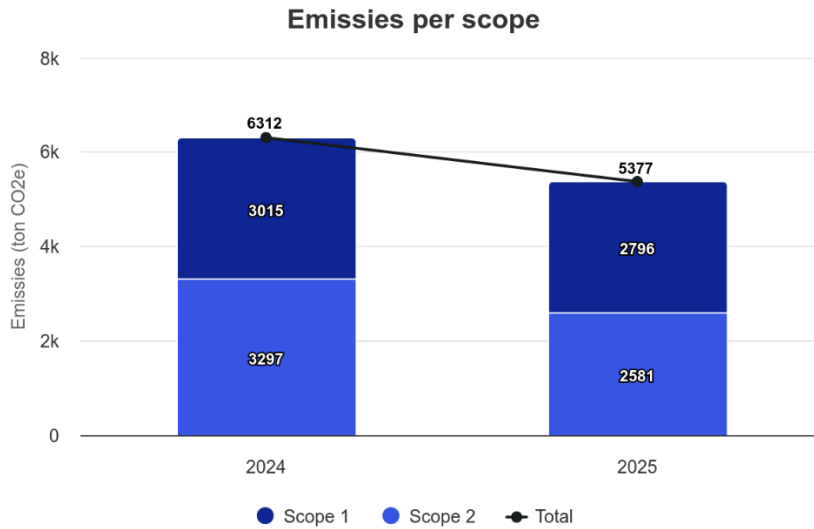
Figuur 3 Scope 1 en 2 CO 2 -emissies van TABS Holland per jaar, locatie-gebaseerd
