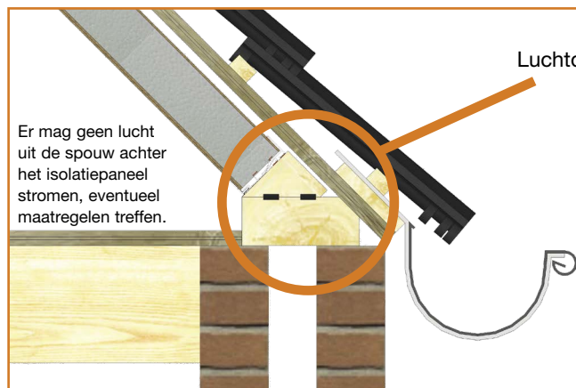
Voetdetail
