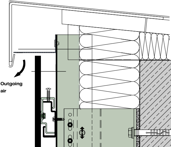
Fascia A109
