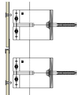
Aluminium achterconstructie met gesloten horizontale voeg
