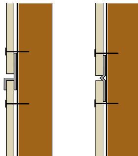
Houten achterconstructie met gesloten en semi-gesloten horizontale voeg
