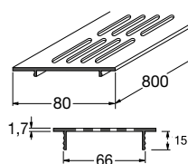
Ventilatieroosters
