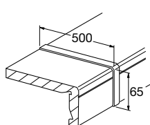
Vensterbank- verbindingsprofielen
