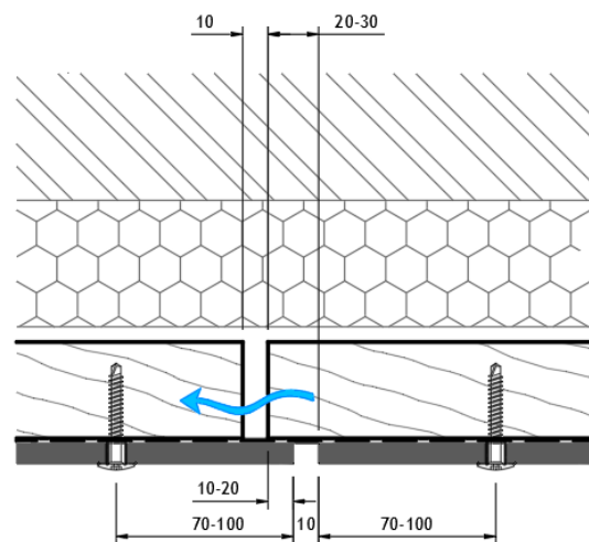
Horizontale doorsnede over plafond
