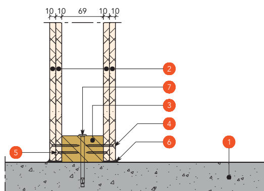
ONDERDETAIL
