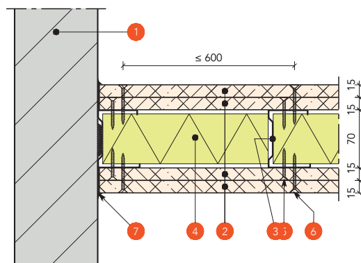
ZIJDETAIL
