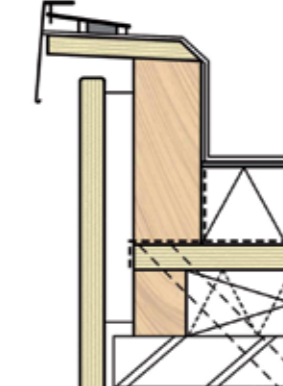
Figuur 8. Voorbeeld uitvoering van een dakoverstek.
