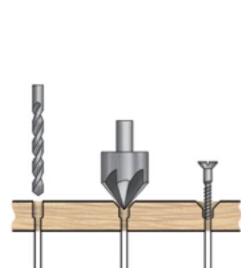
Figuur 2. Schroefgaten in de plaat voorboren met een diameter gelijk aan de steel van de schroef. Vervolgens met een verzink- of soeverreinboor de schroefkop verzinken.
