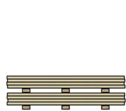
Figuur 1. De platen op een vlakke ondergrond met voldoende ondersteuning opslaan. Bij meer pakketten de balkjes recht boven elkaar plaatsen.
