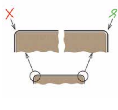
Figuur 5. Rond de randen af met minimaal R3, hierdoor dekt de verflaag in gelijke laagdikte. Bij een niet-afgeronde rand komt er nauwelijks verf op de scherpe rand.
