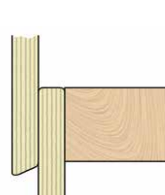
Figuur 6. Goed uitgevoerde horizontale naad met afschuining.
