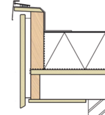
Figuur 9. Voorbeeld aanbrengen van een boeiiboord.
