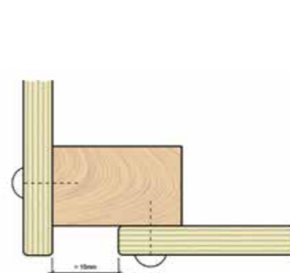
Figuur 4. Goed uitgevoerde hoekaansluiting met voldoende dilatatie.
