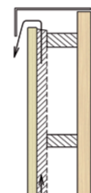
Figuur 3. Schematische voorstelling van de juiste wijze van ventileren.
