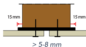
Houten draagconstructie, verticale voegoplossing met EPDM voegband
