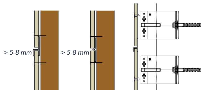
Houten draagconstructie met een gesloten (links) en semi-gesloten (rechts) horizontale voeg
