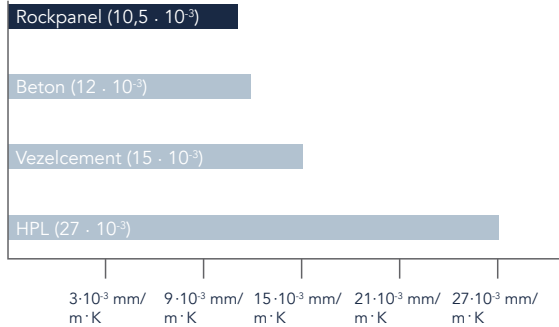
Lineaire uitzettingscoëfficiënt
