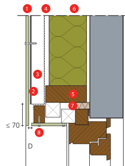
1-351 | mechanische bevestiging op hout, bovenaansluiting venster
