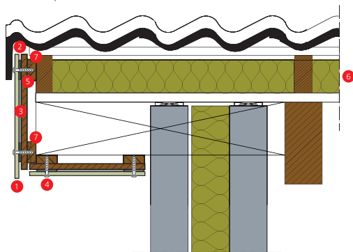
1-511 | mechanische bevestiging op hout, dakoverstek renovatie
