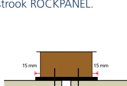
Houten draagconstructie, verticale voegoplossing
