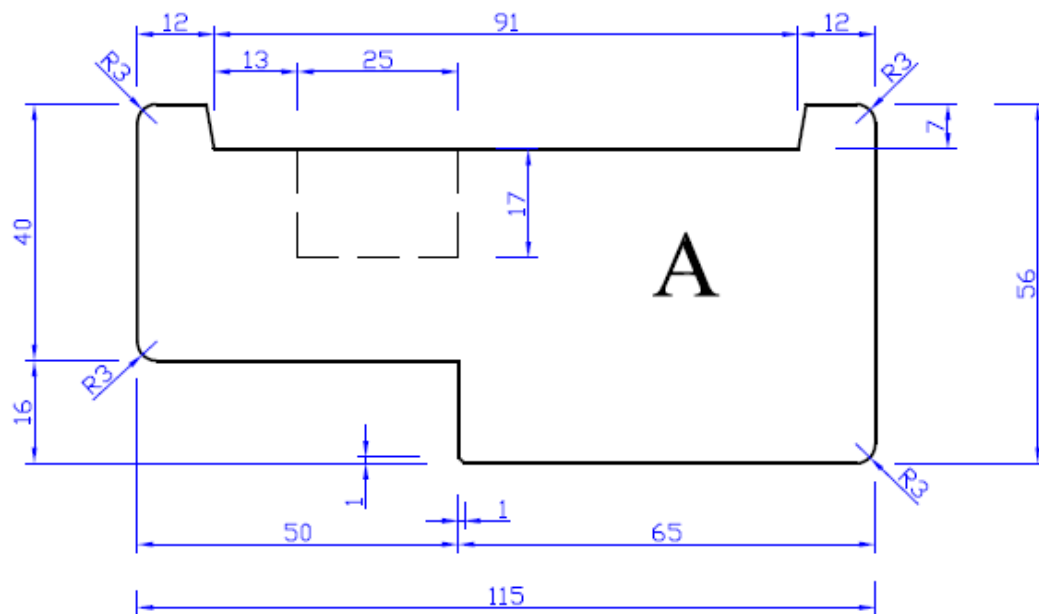
Bovendorpel
