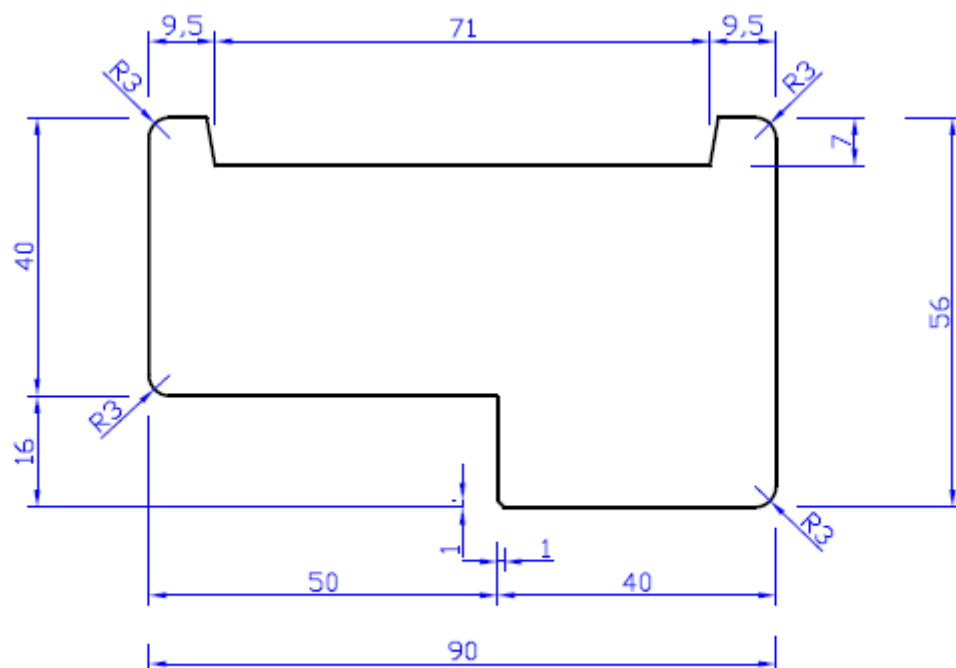
Bovendorpel
