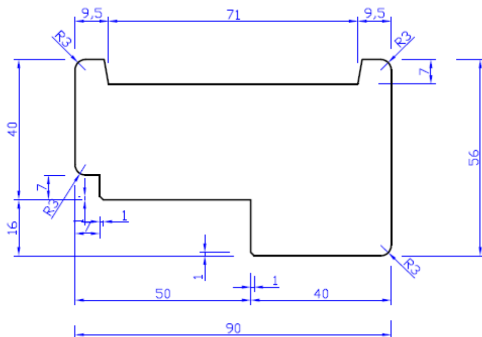
Stijl
