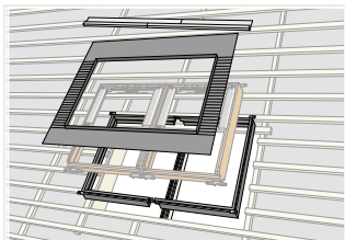
18 mm gekoppeld met EBY ondersteuningsbalk BDX -K-- 2011
