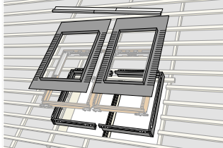
100 mm gekoppeld met EKY ondersteuningsbalk BDX -K- 2011E
