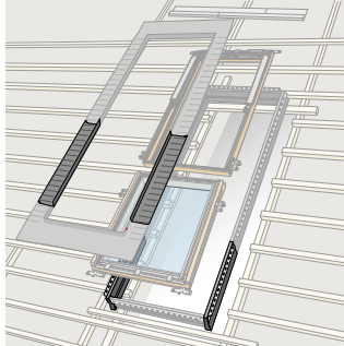
Montage met verlengstuk voor GIU/GIU of GDL BDX WK34 2000 Bij verdiepte montage BDX -K-- 2000F
