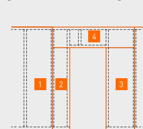
Deuropening bij horizontale beplatingsvoeg
