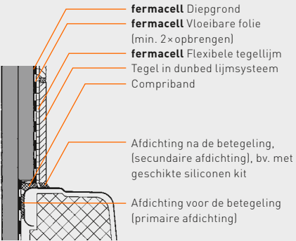
Aansluiting aan Powerpanel H 2 O-montagewand met doorgaande éénlaagse Powerpanel H 2 O beplating en dubbele beplating boven de badkuip
