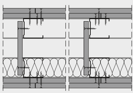
Verbinding bij een installatiewand
