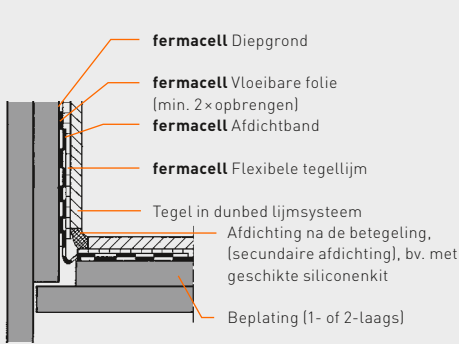
Aansluiting wandhoek in een omgeving met waterbelasting
