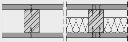
Montagewand met/zonder isolatie van de holle ruimte, uitgevoerd als enkelvoudige staanderwand met éénlaagse beplating
