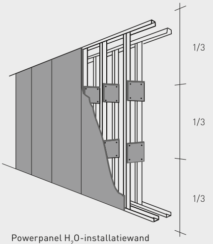
Powerpanel H 2 O-installatiewand
