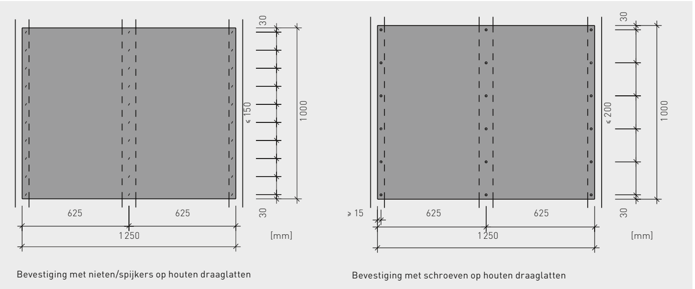
Hartafstand van de draaglatten en afstand van de verbindingsmiddelen bij geventileerde vliesgevels
