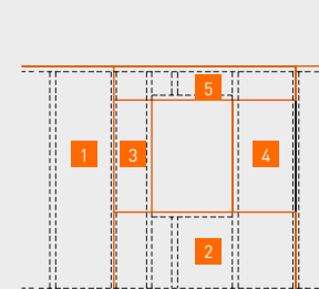
Raamopening bij horizontale beplatingsvoeg
