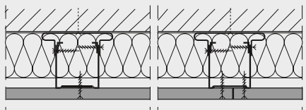
Onderconstructie uit CW-profiel met verende aanpasbeugel, éénlaagse beplating
