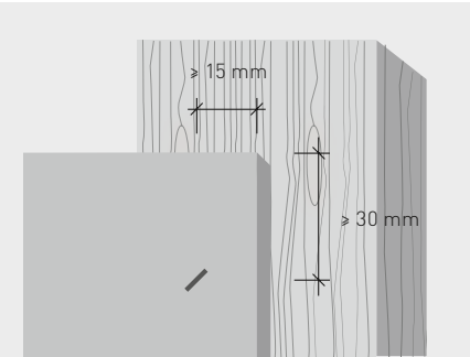
Randafstanden Bij gebruik van schroeven, hechtnieten of spijkers moet een voldoende grote minimum-afstand van ≥ 15 mm of ≥ 30 mm tot de plaat-rand worden bewaard.
