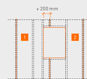
Raamopening met plaatuitspringing (variant A)
