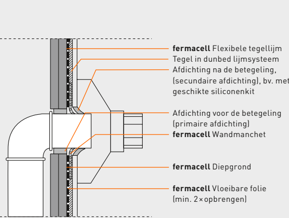
Doorvoer door Powerpanel H 2 O-montagewand
