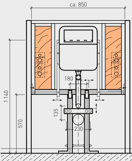
Draagstaanders voor hangtoiletten met inbouwreservoir en de mogelijkheid van ondersteuning van draagarmen (maten in mm)
