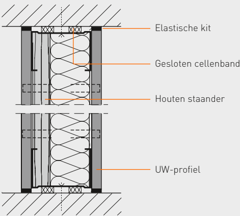
Plafond- en vloeraansluiting
