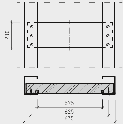
Houten plank of spaanplaat voor kleine wastafels (maten in mm)
