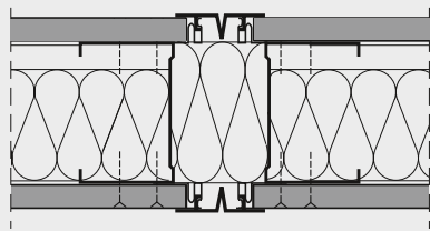
fermacell Powerpanel H 2 O-montagewand, dilatatievoeg met extra profiel (geen brandeis)
