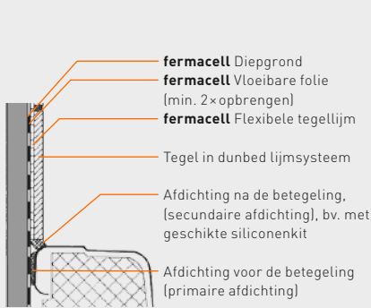
Wandaansluitingen van douche- of badkuipen, aansluiting aan Powerpanel H 2 O-montagewand met één beplatingslaag
