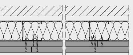
Powerpanel H 2 O-voorzetwand, tweelaagse beplating
