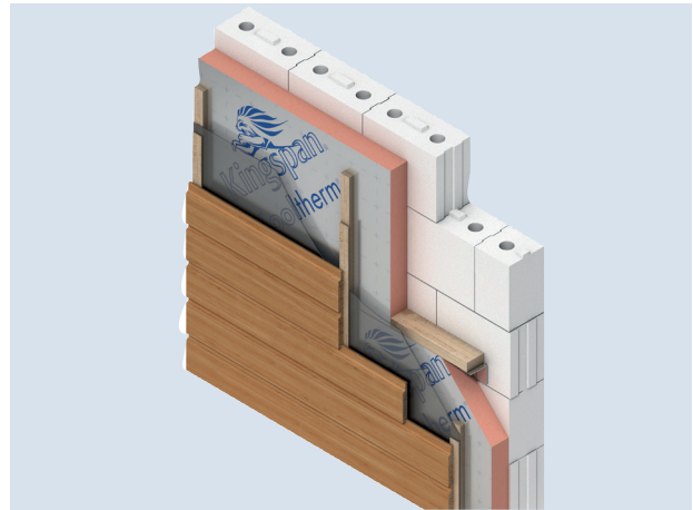
R c -waarden bij toepassing van verschillende diktes Kingspan Kooltherm ® K12 Frameplaat bij verschillende houtpercentages
