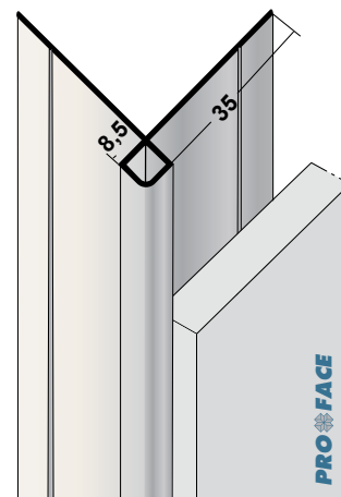
Proface®-CORNEX C85-A
