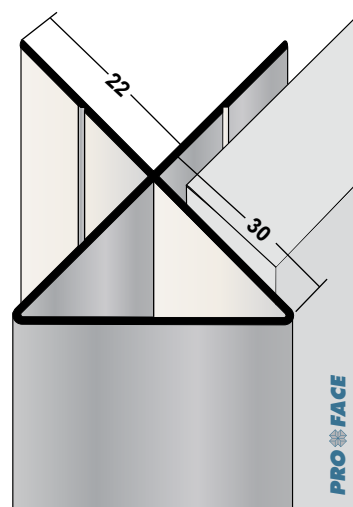
Proface®.CORNEX C300-A
