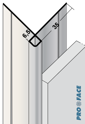
Proface®-CORNEX C65-A
