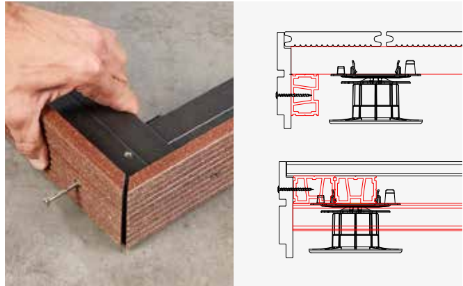
Afwerking met randplank (links) en Afdekstrip Piazza (rechts)
